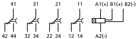
Schema Attrazione RDT.x4c-x9c
