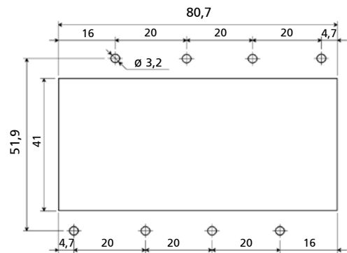
Dima di foratura
