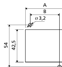
Dima foratura
