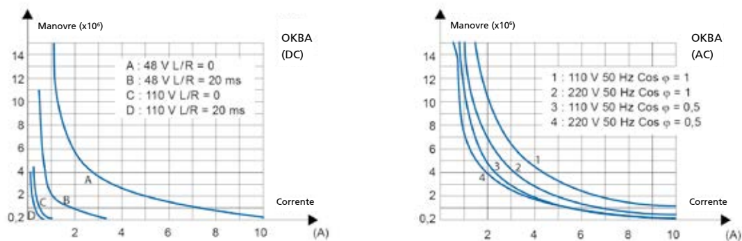
OKBA: altri esempi di vita elettrica disponibili dalla scheda tecnica del relè serie OK (modello OKSFC)
