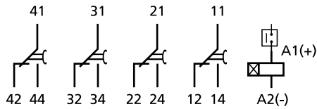
Schema Attrazione RDT.x1c-x7c
