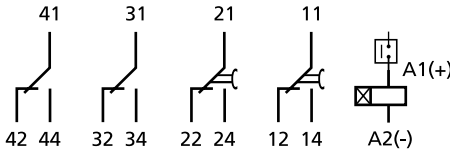
Schema Attrazione RDT.x2c-x8c
